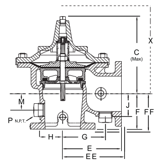
2100GS (Angle)
