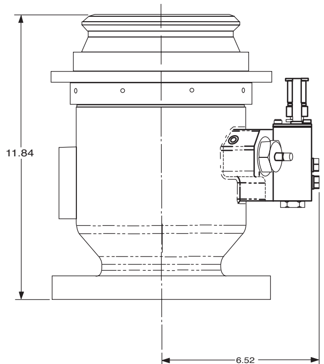
外部尺寸图 (inches)
